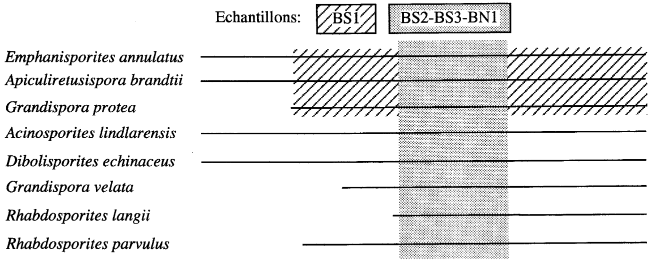
Figure 11: Position stratigraphique des principales espèces de spores provenant des grès verts de la carrière Brandt sud (BS) et des grès blancs de la carrière Brandt nord (BN).
