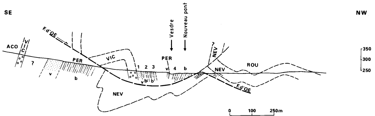
Figure 10: Coupe géologique de la vallée de la Vesdre à Membach. 1 à 4: barres grésos-conglomératiques kaolineuses. Pour la signification des sigles de formation, se reporter à la figure 2.
