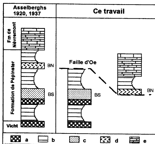
Figure 3: Colonne stratigraphique schématique de la Formation de Pépinster à Goé d'après d'Asselberghs (1920, 1937), confrontée à l'interprétation retenue dans ce travail. a. conglomérats; b. siltites et shales bordeaux; c. grès verts; d. grès blancs; e. calcaires.
