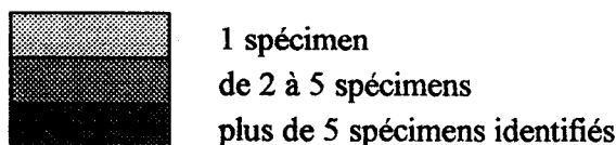
Figure 12 : Répartition des macrorestes végétaux en fonction des différents gisements.
