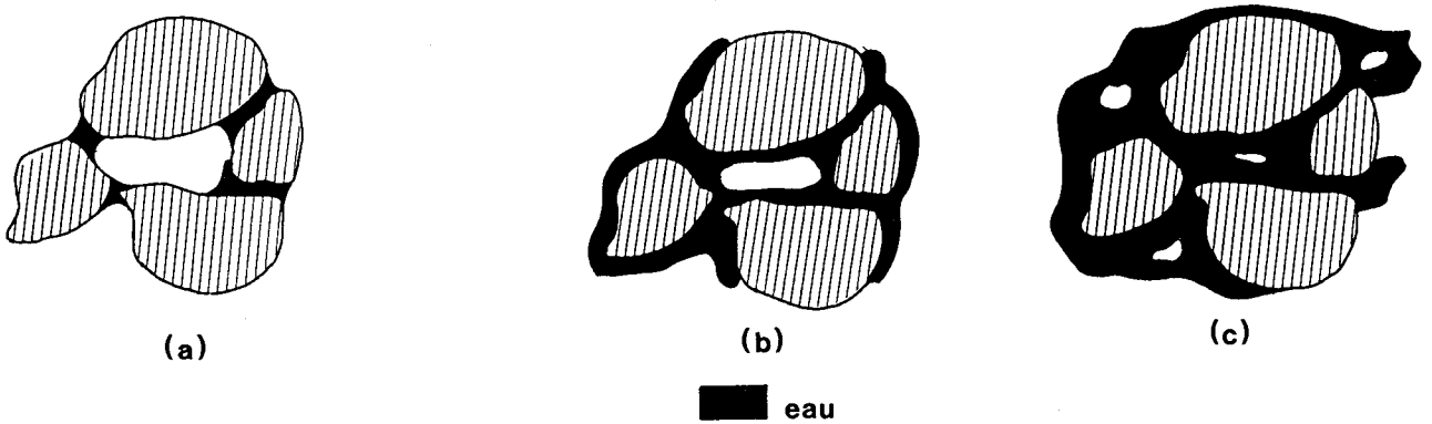
Fig. 4. Répartitions de l'eau et de l'air à différentes saturations : a) formation de ménisques à faible saturation, b) augmentation de la saturation en eau, c) bulles d'air piégées correspondant à une saturation résiduelle en air.
