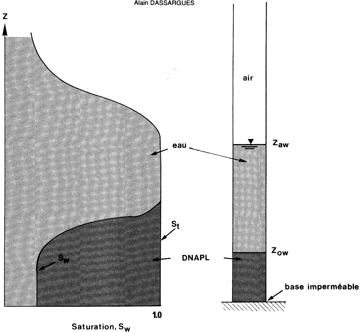
Fig. 13. Profil vertical des saturations et hauteurs piézométriques, obtenues pour un système air-eau-DNAPL.
