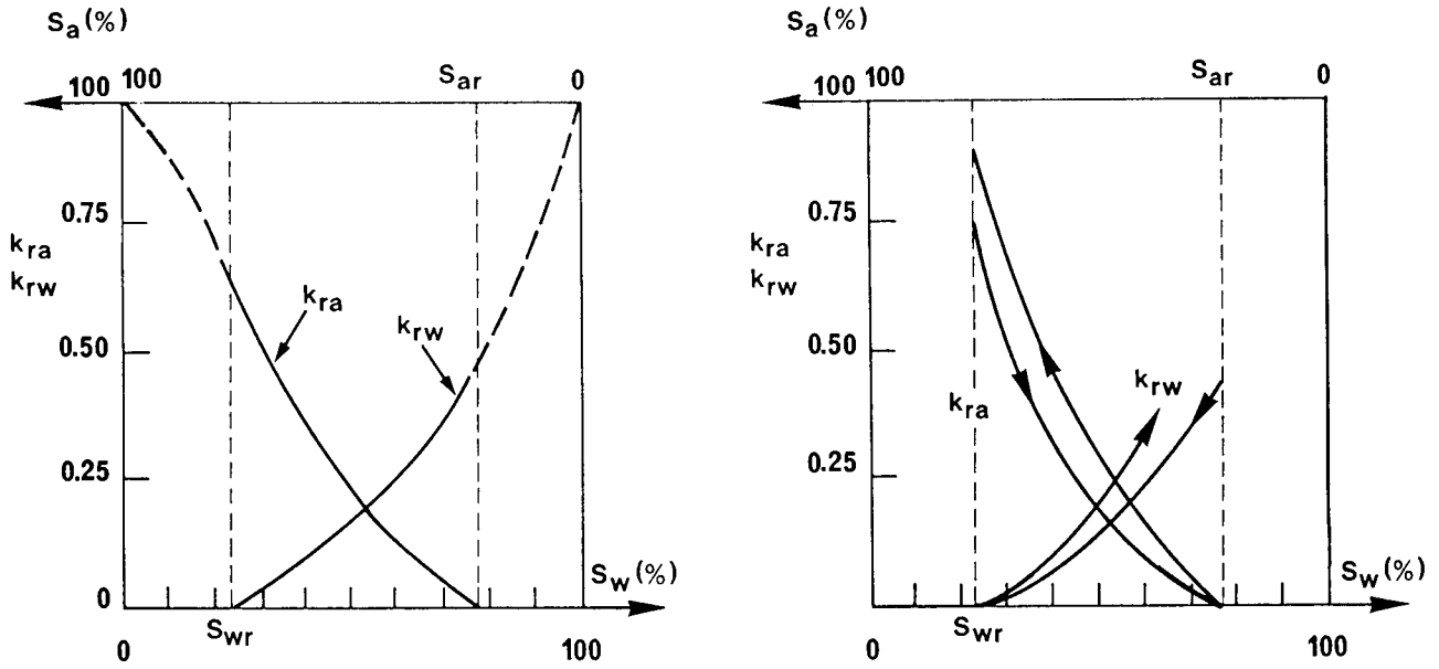
Fig. 14. Courbes de perméabilités relatives typiques: (a) sans hystérésis, (b) avec hystérésis.
