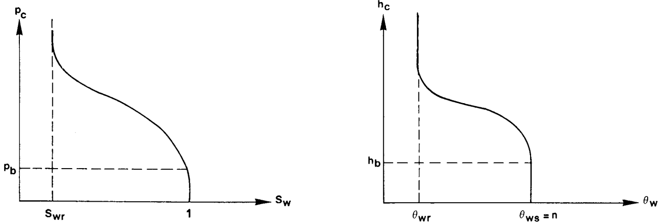
Fig. 6. Courbe de rétention.
