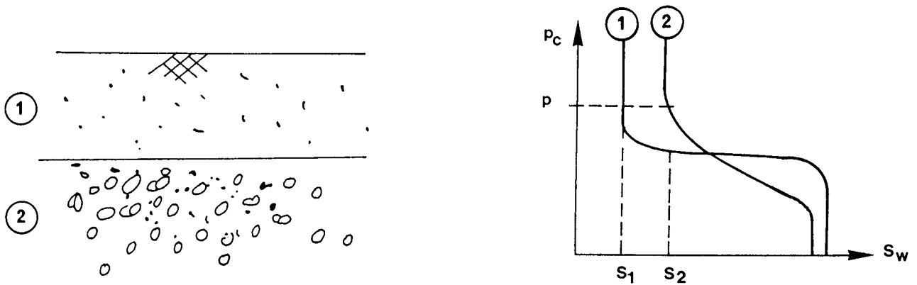
Fig. 9. Discontinuité de la saturation à une pression capillaire donnée (p), à l'interface entre 2 milieux poreux.
