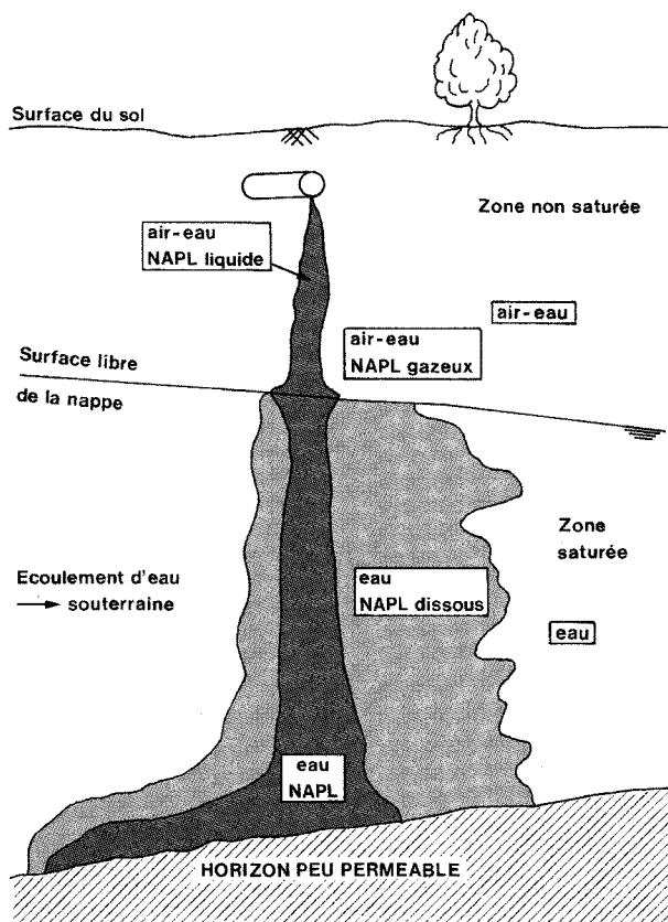
Fig. 16. Même situation qu'à la figure 15 mais le liquide est plus dense que l'eau (d'après Celia et al. , 1993).
