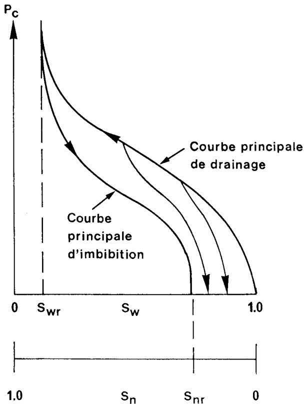
Fig. 7. Hystérésis des courbes de pression capillaire.
