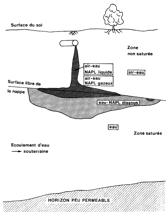
Fig. 15. Situation typique de pollution des zones saturée et non saturée par un produit liquide non aqueux formant une phase séparée ("NAPL"), cas où le liquide est moins dense que l'eau (d'après Celia et al. , 1993).
