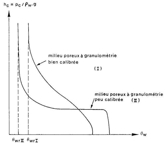
Fig. 5. Courbes typiques de la pression capillaire en fonction de la teneur en eau.
