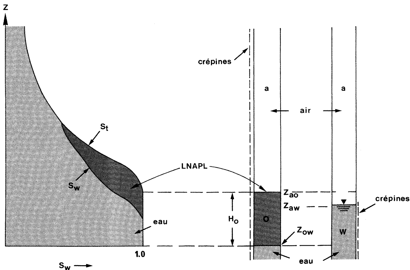
Fig. 12. Profil vertical des saturations et hauteurs piézométriques, obtenues pour un système air-eau-LNAPL.
