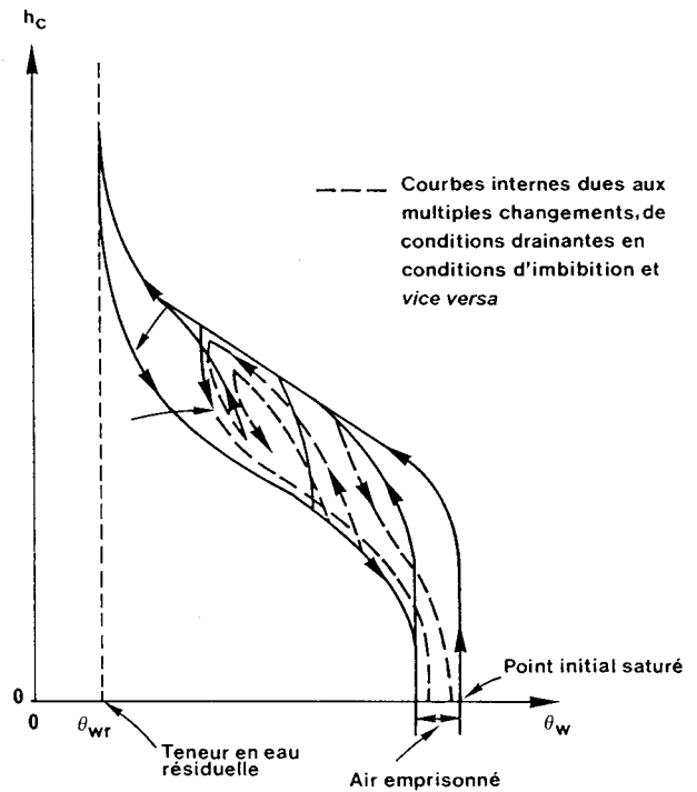
Fig. 8. Hystérésis multiples (d'après Bear, 1993).
