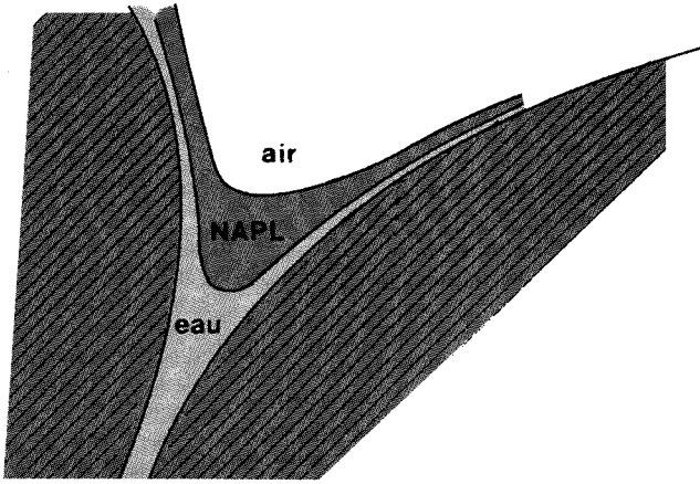
Fig. 11. Image d'un pore du milieu avec les 3 phases fluides.
