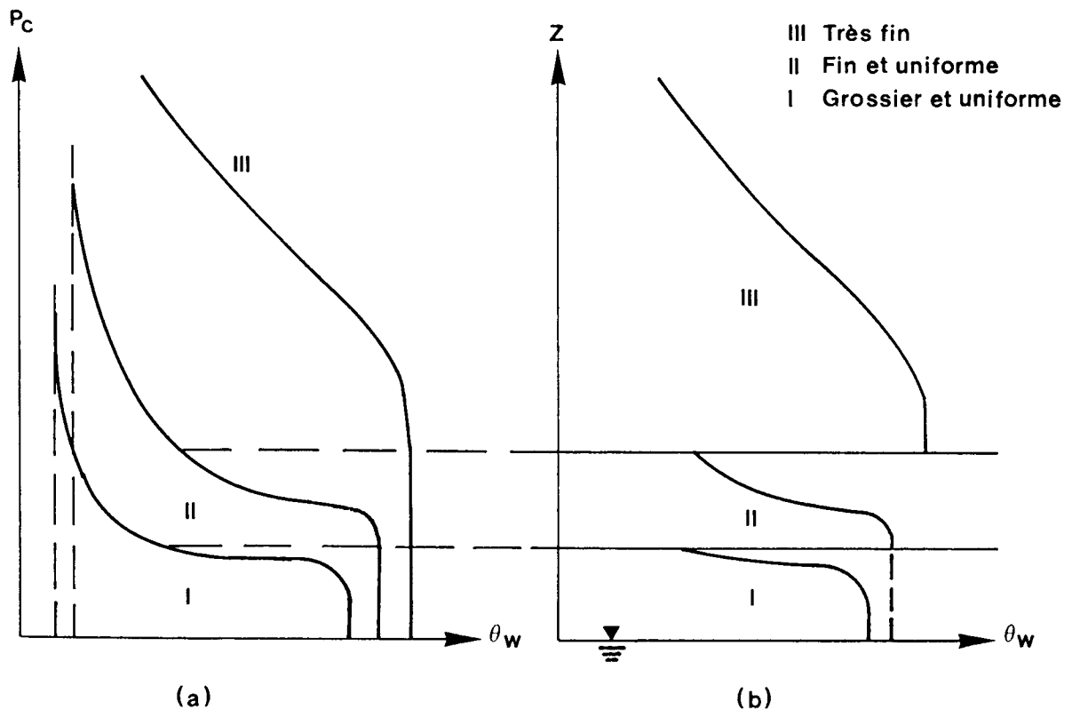
Fig. 10. Sauts de saturation en conditions statiques: (a) courbes de pression capillaire pour les 3 sols, (b) profil vertical de la saturation ou de la teneur en eau dans un système à 3 couches (d'après Bear, 1993).
