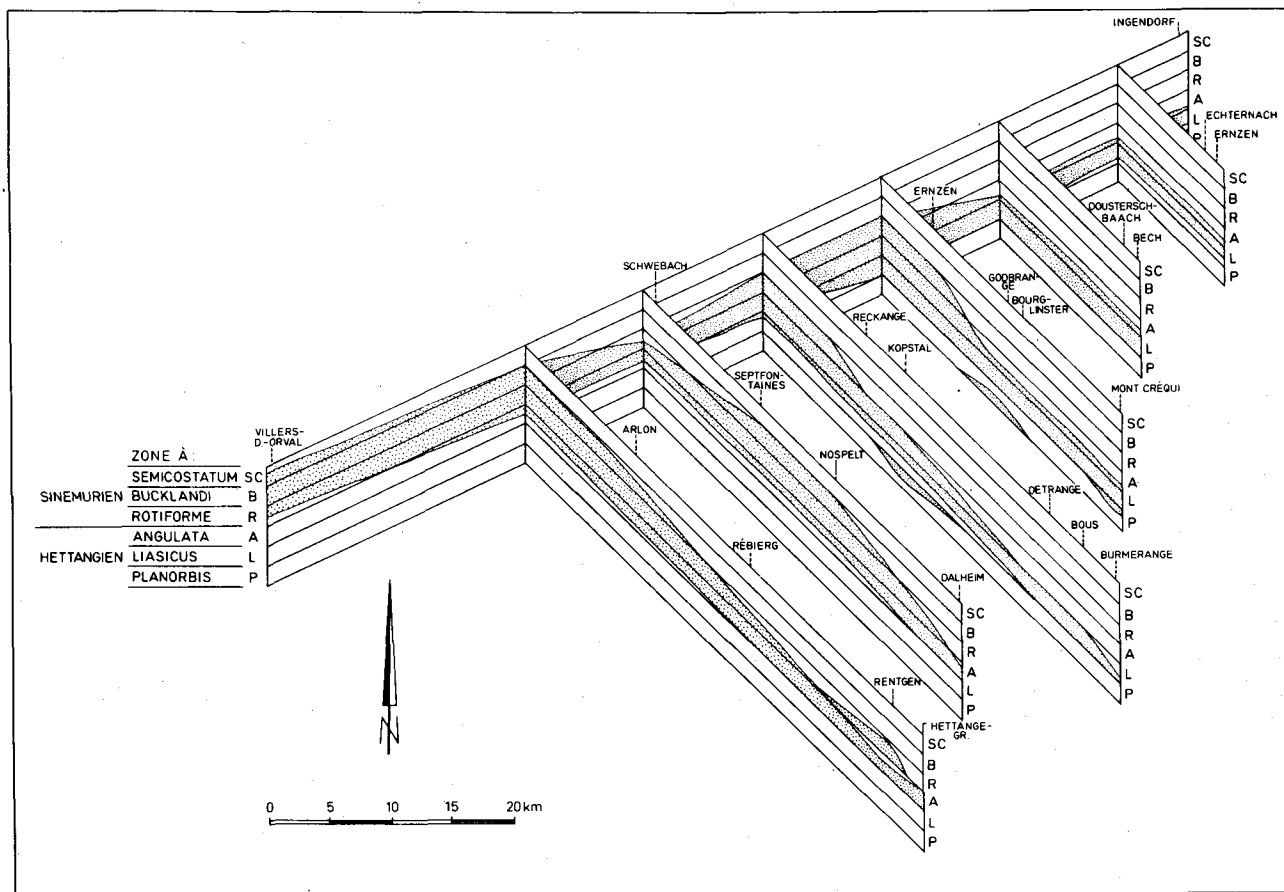
FIG. 2.- Les Grès du Luxembourg (en pointillé), au Luxembourg et dans les régions voisines : diachronie de la formation par rapport aux biozones de l'Hettangien et du Sinémurien.
