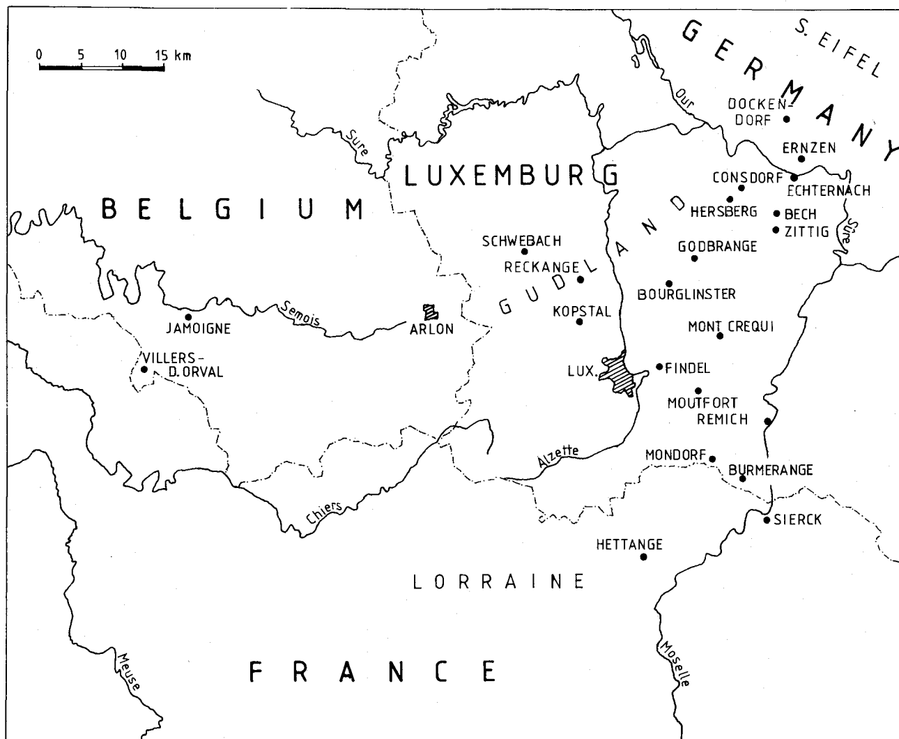
FIG. 1.- Situation des principaux gîtes fossilifères dans l'Hettangien du NE du Bassin de Paris.
