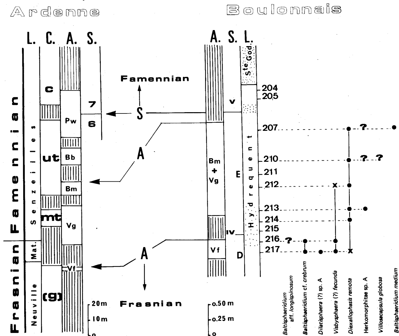
Figure 2.- Comparaison entre l'Ardenne et le Boulonnais à la transition Frasnien-Famennien.
