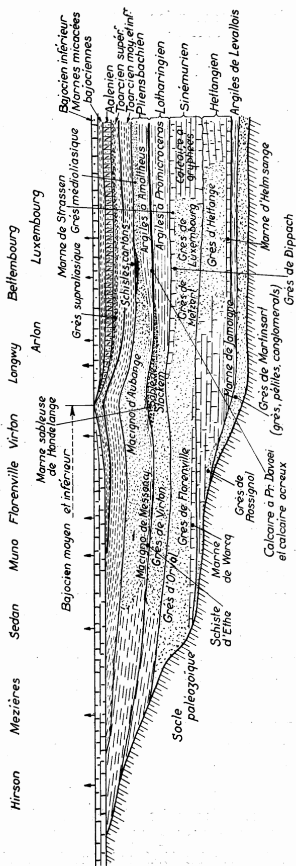
FIG. 4. — Coupe schématique à travers le Lias belgo-luxembourgeois suivant une direction est-ouest. (D'après VAN WERVEKE et LUCIUS, très modifié).
