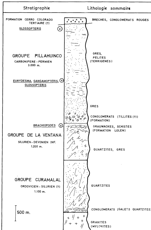
Fig. 3. — Stratigraphie des formations sédimentaires de la chaîne de la Ventana.
